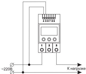
Схема подключения
