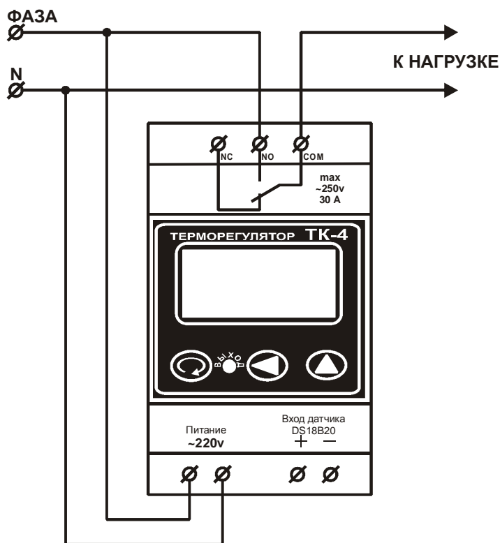
Рис.1 Схема подключения терморегулятора ТК-4
