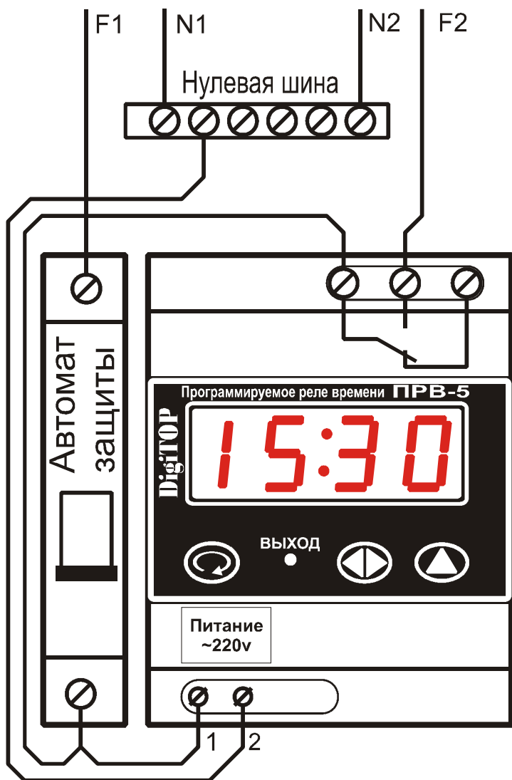
Рис.1 Монтажная схема реле времени
